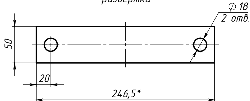
Поз.4 (Полухомут) развертка
