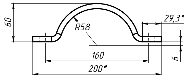
Поз.4 (Полухомут)
