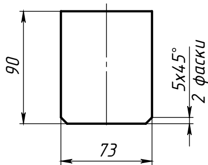
Поз.3 (Ребро среднее)
